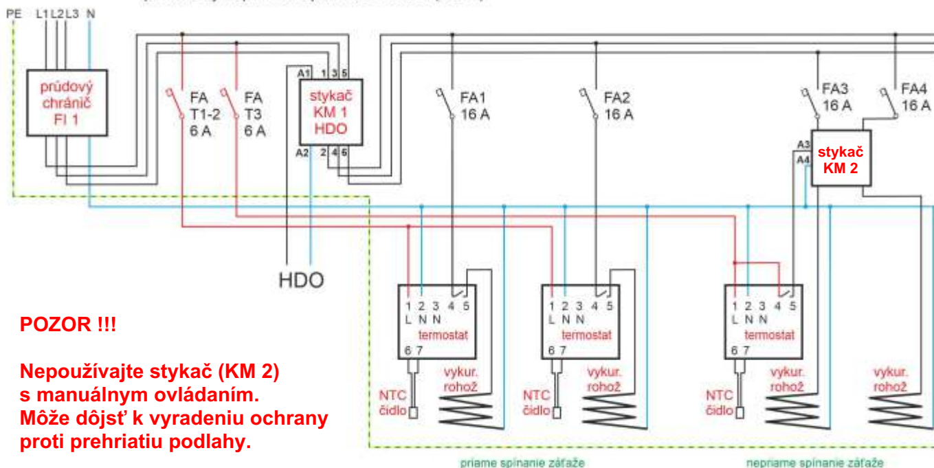
Principiálna schéma zapojenia termostatov priame aj nepriame spínanie záťaže (HDO)
